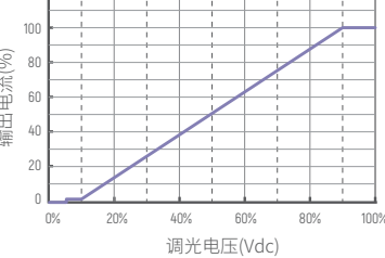
PWM曲线
