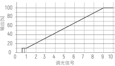
调光曲线
