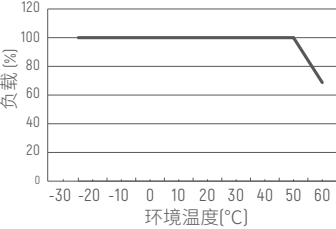
降额曲线
