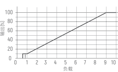
调光曲线
