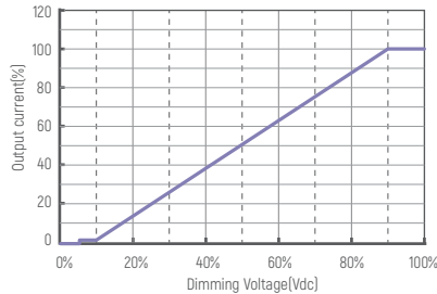
PWM曲线
