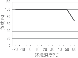
降额曲线
