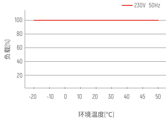
降额曲线
