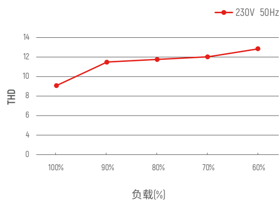
THD vs 负载曲线
