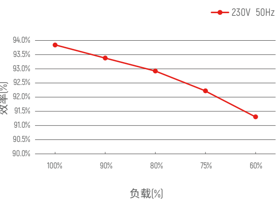
效率 vs 负载曲线
