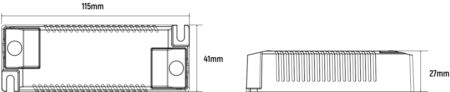
尺寸(mm)
