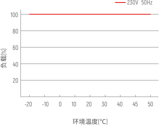
降额曲线
