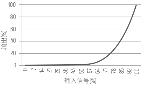
调光曲线
