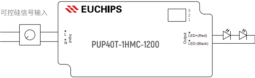
应用连接图
