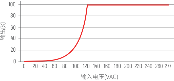
调光曲线
