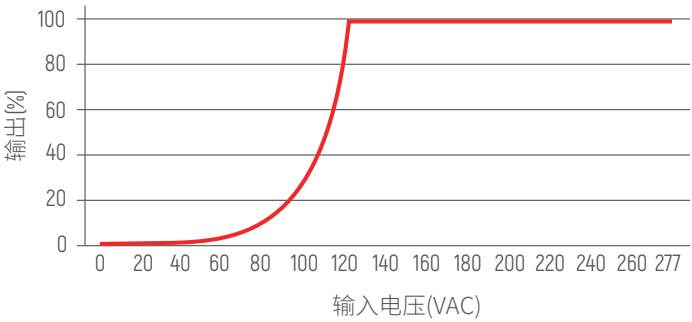
调光曲线
