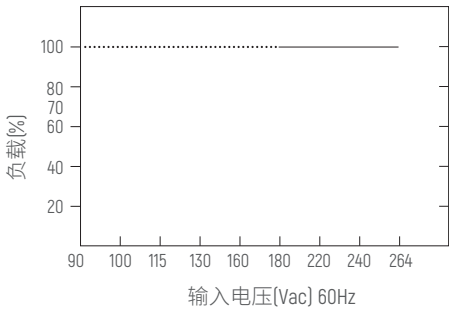
静态特性曲线
