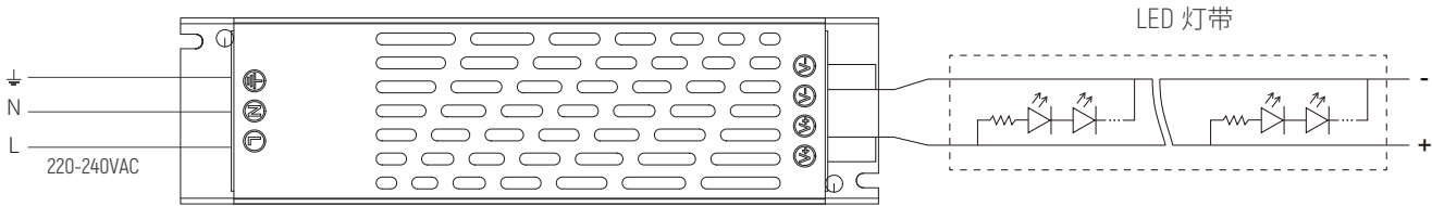
接线图
