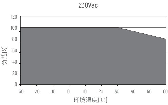
降额曲线
