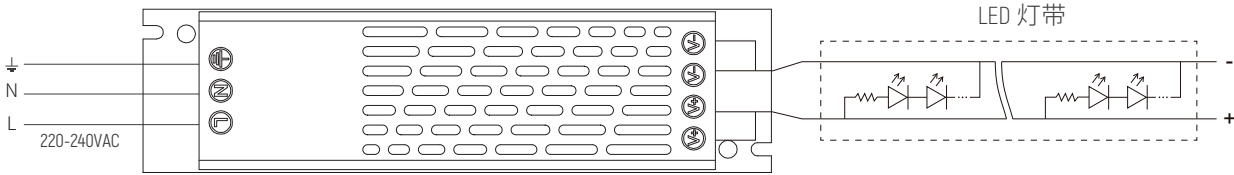
接线图
