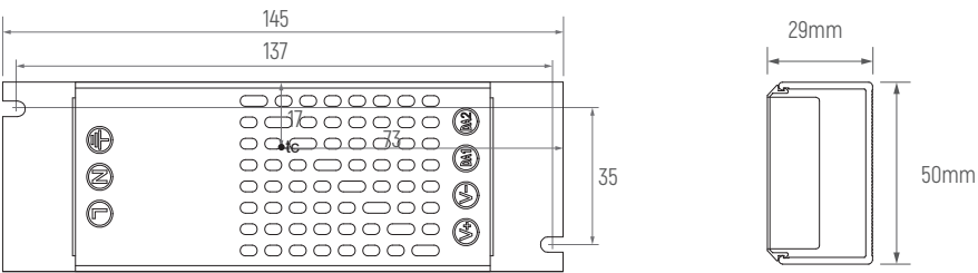
尺寸(mm)
