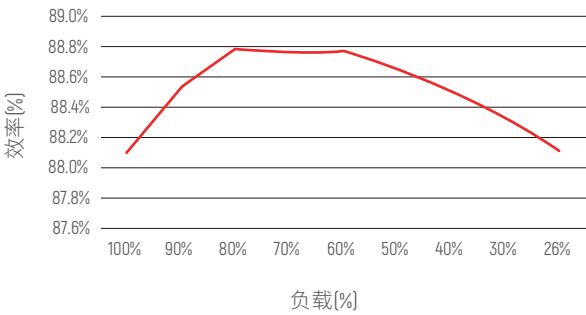
效率曲线
