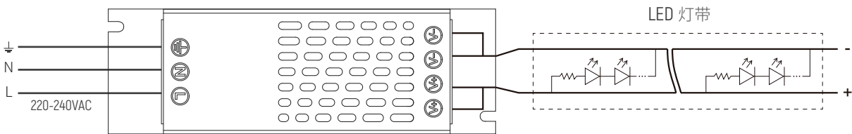
接线图
