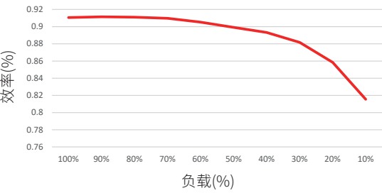
效率 Vs 负载
