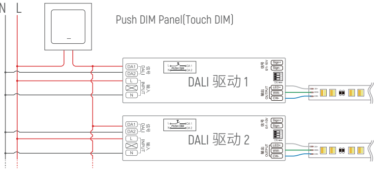
Push DIM (Touch DIM)应用图
