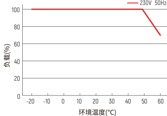
降额曲线
