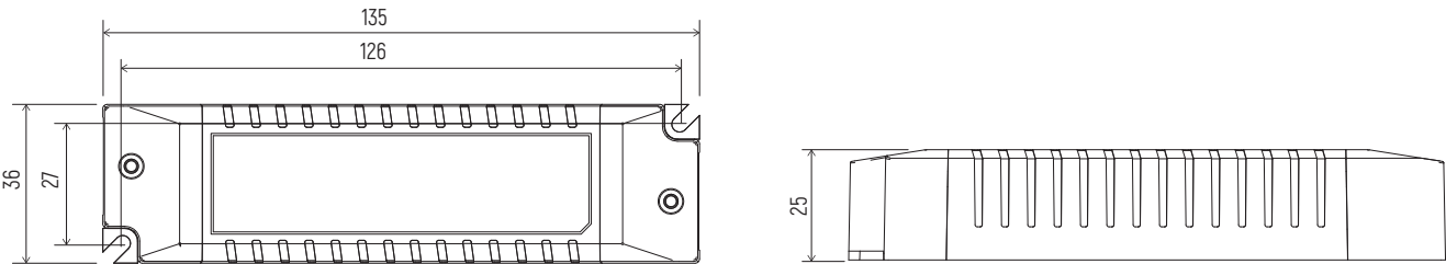
尺寸图(mm)
