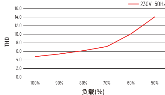
THD vs 负载曲线
