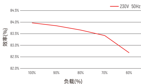
效率 vs 负载曲线
