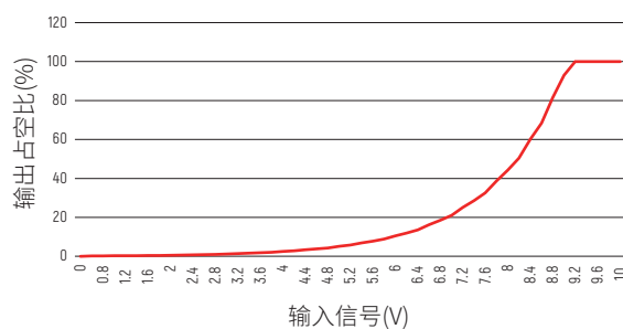
0/1-10V 曲线
