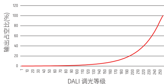
DALI 曲线
