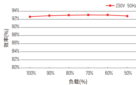
效率 vs 负载曲线
