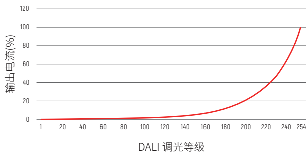
DALI 曲线
