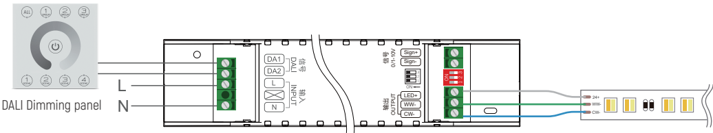
DALI Wiring
