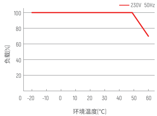
降额曲线
