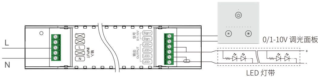
接线图
