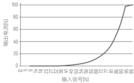
调光曲线图
