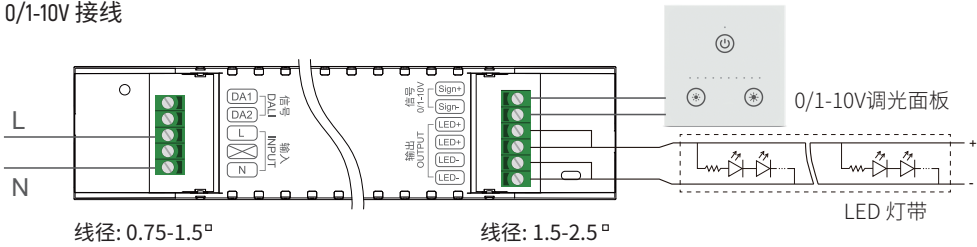
0/1-10V 接线
