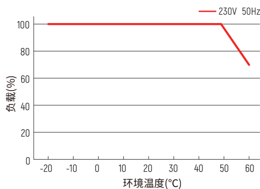
降额曲线
