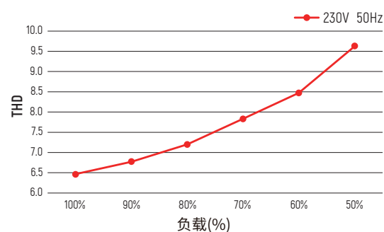
THD vs 负载曲线
