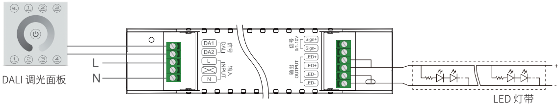
DALI 接线
