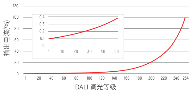
DALI 曲线
