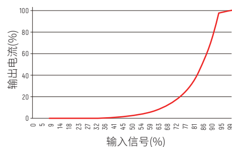
0/1-10V 曲线
