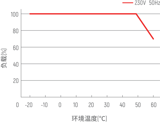
降额曲线
