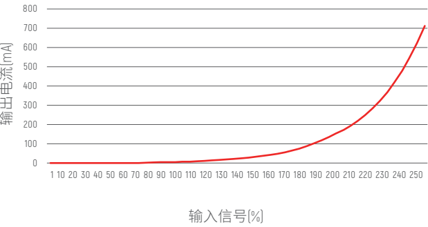
DALI 曲线
