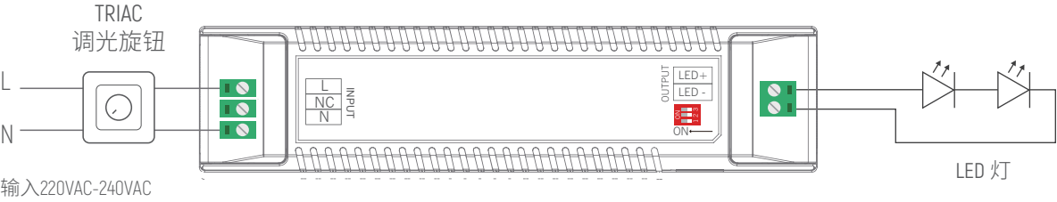
接线图
