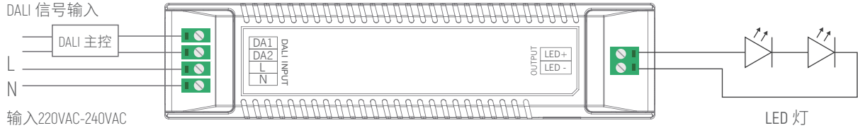
接线图
