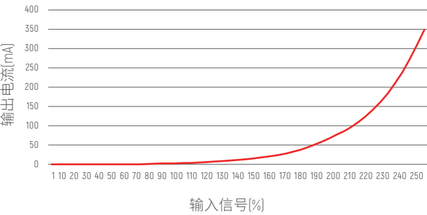
DALI 曲线
