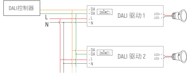
DALI应用接线图
