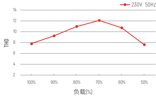
THD vs 负载曲线
