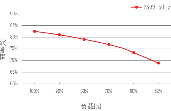
效率 vs 负载曲线
