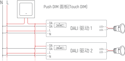
Push DIM(Touch DIM) 接线图
