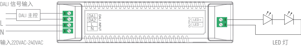
接线图
