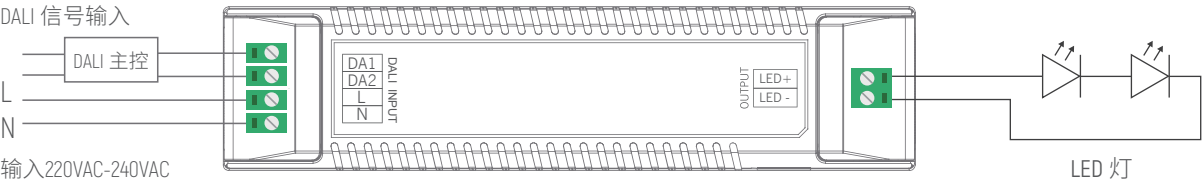
接线图
