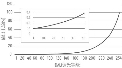
调光曲线
