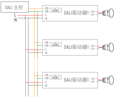
DALI接线图
