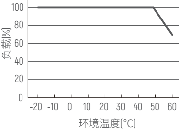
降额曲线
