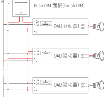
Touch DIM(Push DIM) 接线图
