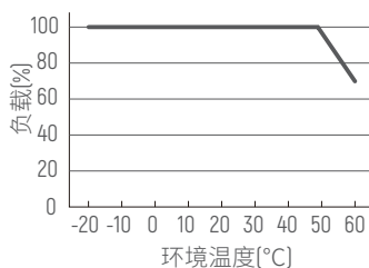
降额曲线
