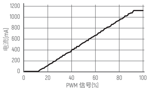
PWM曲线
