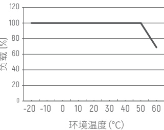
降额曲线
