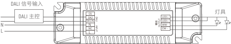
接线图
