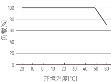
降额曲线
