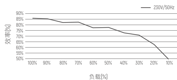
效率曲线
