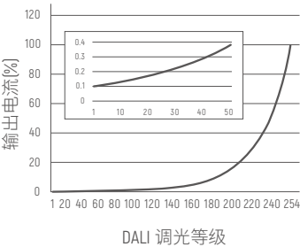
调光曲线
