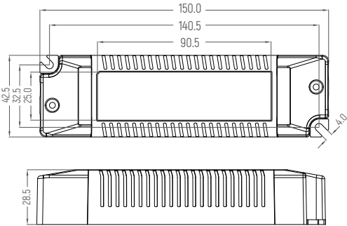
尺寸(mm)
