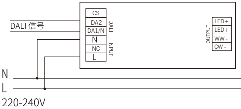
DALI应用图
