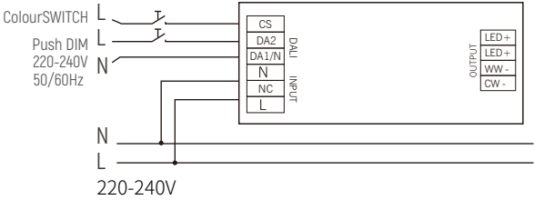
Push DIM (Touch DIM)应用图
