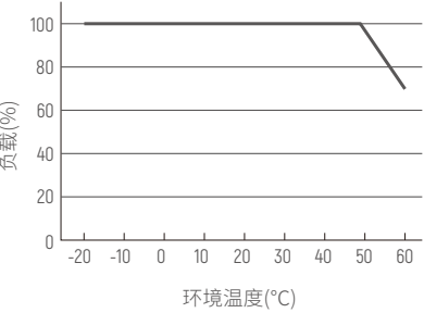
降额曲线
