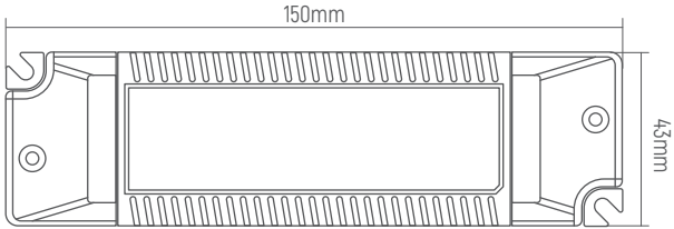
尺寸(mm)
