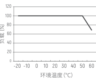
降额曲线
