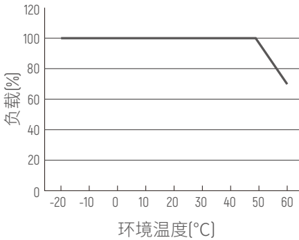
降额曲线
