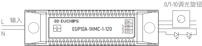
接线图
