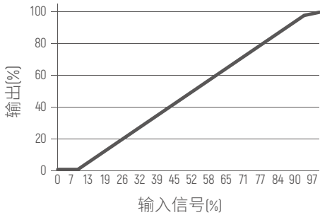
调光曲线
