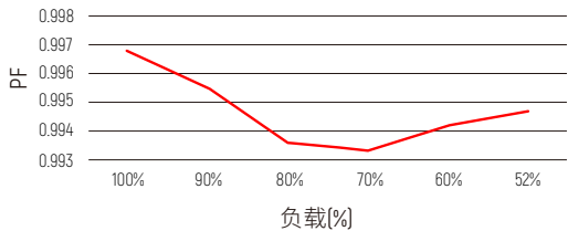
PFvs负载
