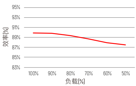
效率vs负载
