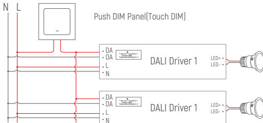
Push DIM (Touch DIM)应用图
