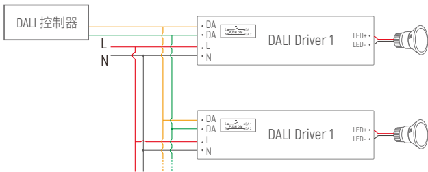
DALI应用图
