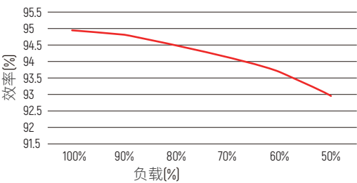
效率 vs 负载
