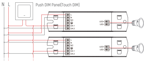
Push DIM (Touch DIM)应用图
