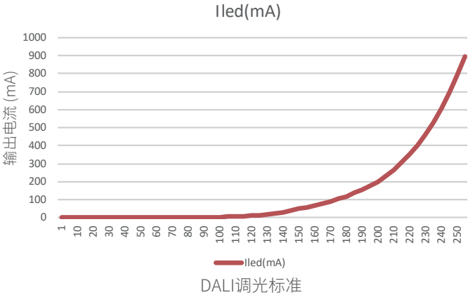
调光曲线
