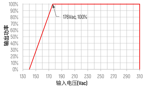
降额曲线
