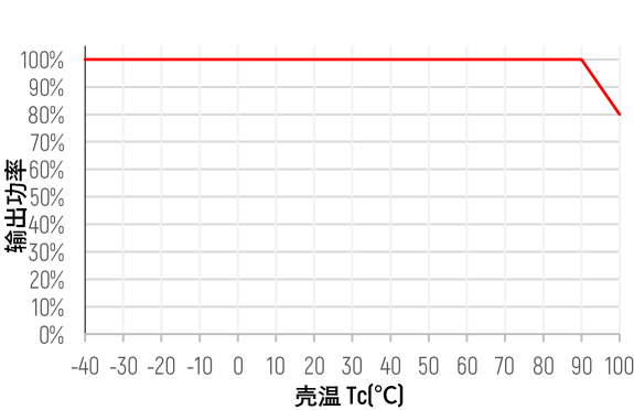
输出功率vs. 壳温
