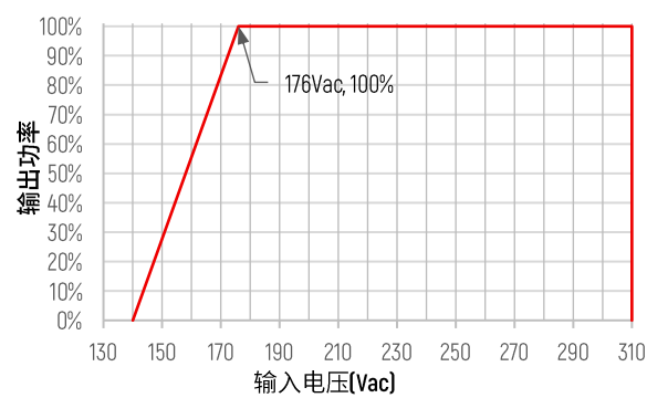
降额曲线
