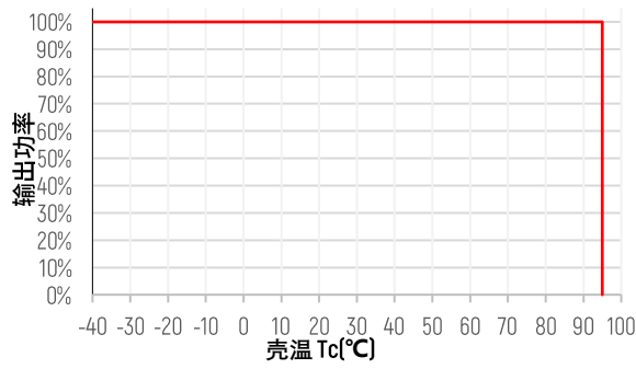
输出功率 vs. 壳温
