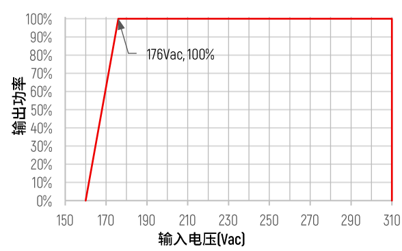
降额曲线
