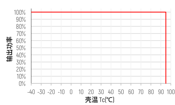
输出功率vs. 壳温
