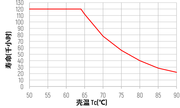
寿命 vs. 壳温
