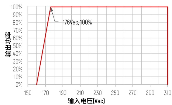
降额曲线
