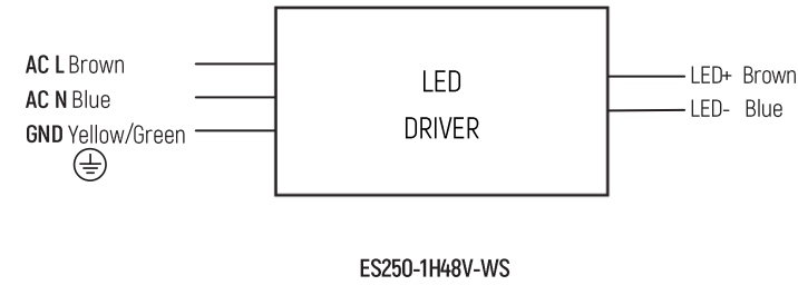
ES250-1H48V-WS
