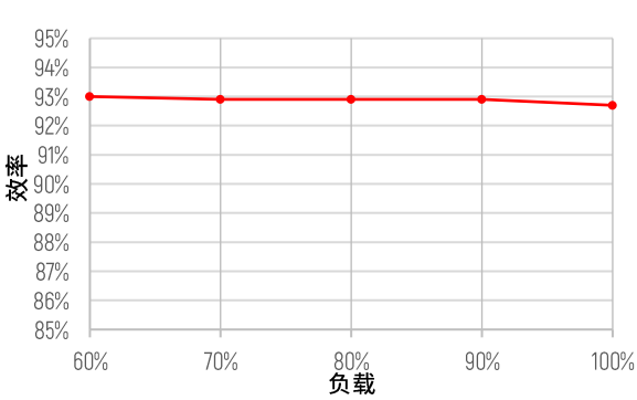
效率vs. 负载
