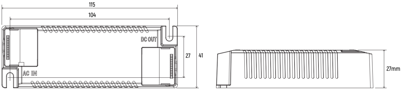
Dimension(mm)
