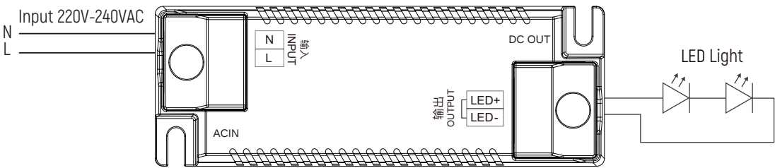
Wiring
