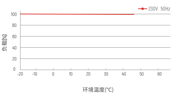
降额曲线
