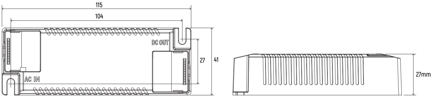
尺寸(mm)
