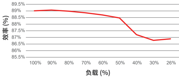
效率曲线
