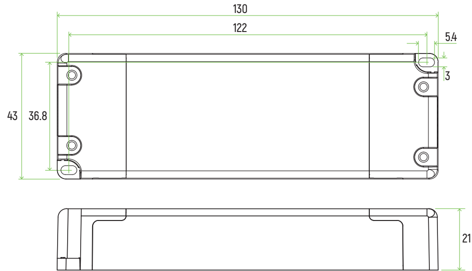
尺寸(mm)
