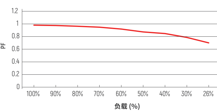
PF曲线
