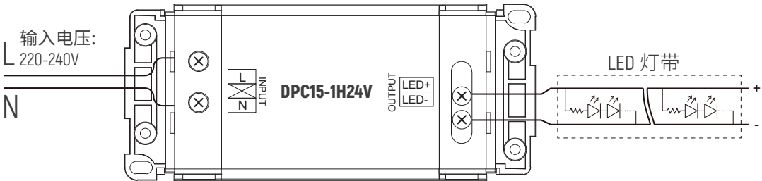
接线
