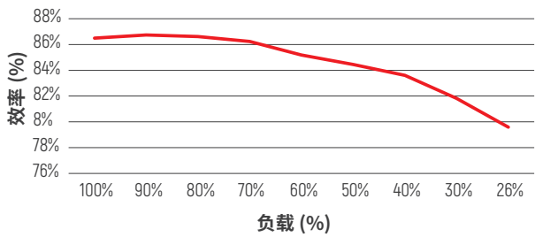
效率曲线
