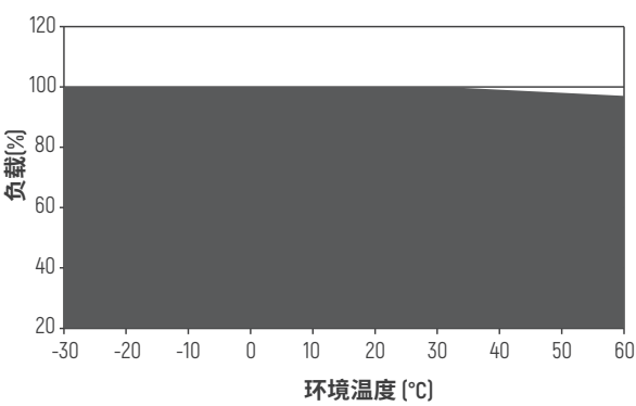
降额曲线
