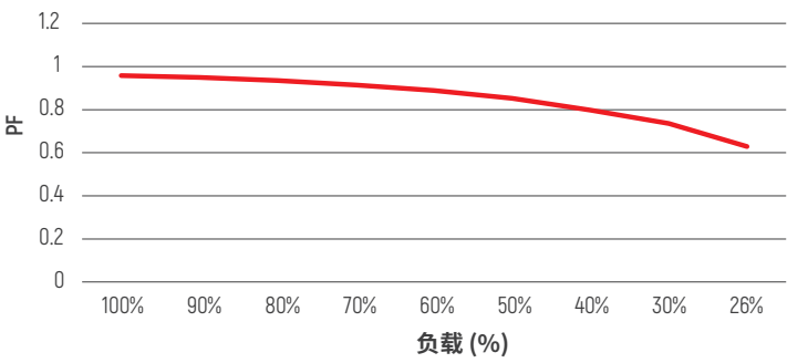
PF曲线
