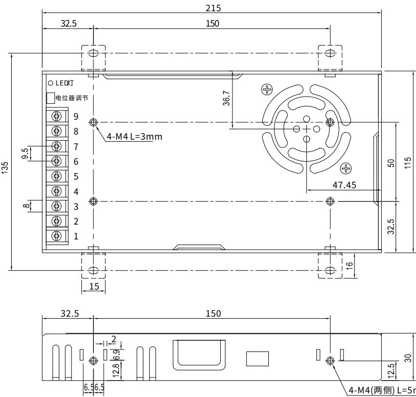
机构尺寸
