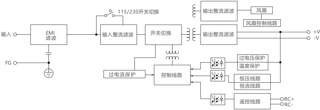
线路框图
