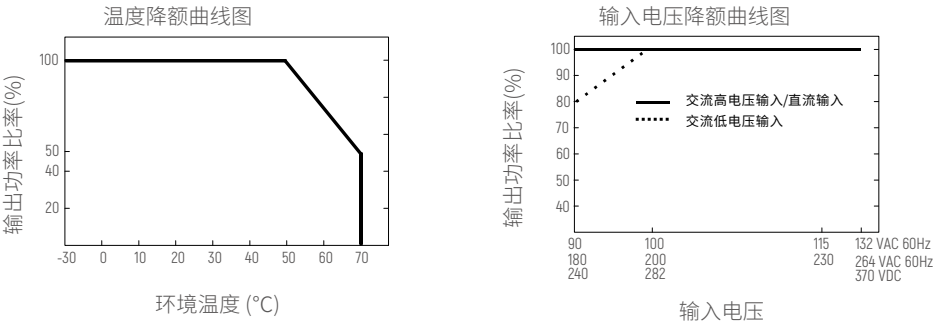
产品特性曲线
