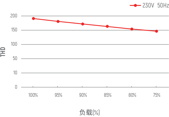
THD vs 负载曲线
