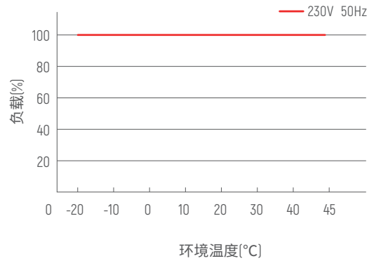
降额曲线
